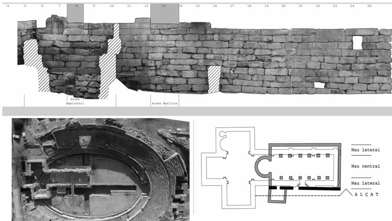
Figura 2 Alçat de la fonamentació de la basílica visigòtica de l'amfiteatre de Tarraco.
