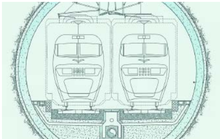
Dibuix del projecte de les vies dins el túnel.
